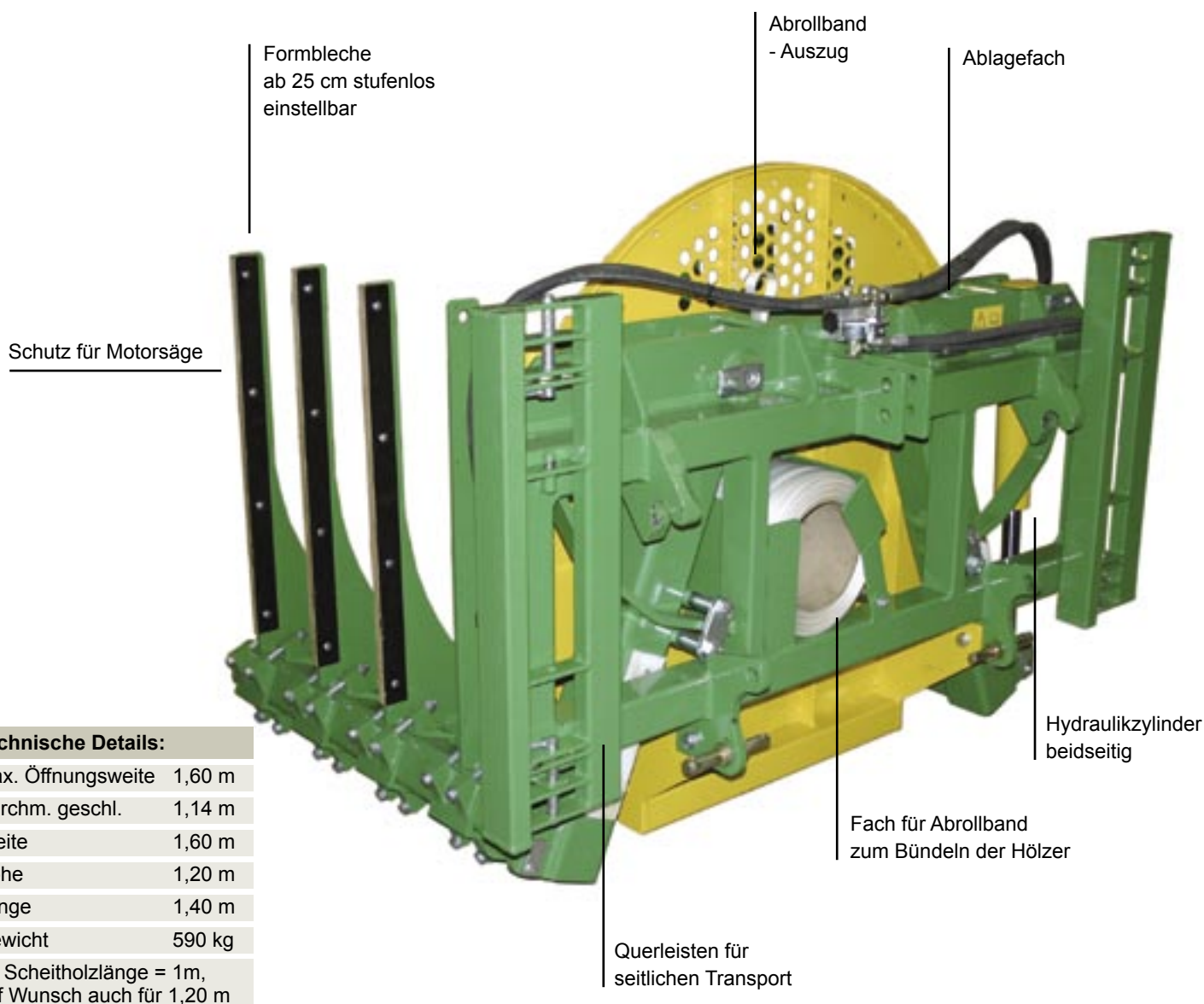
Montage der Querstreben, um das Bündel seitlich zu packen.
